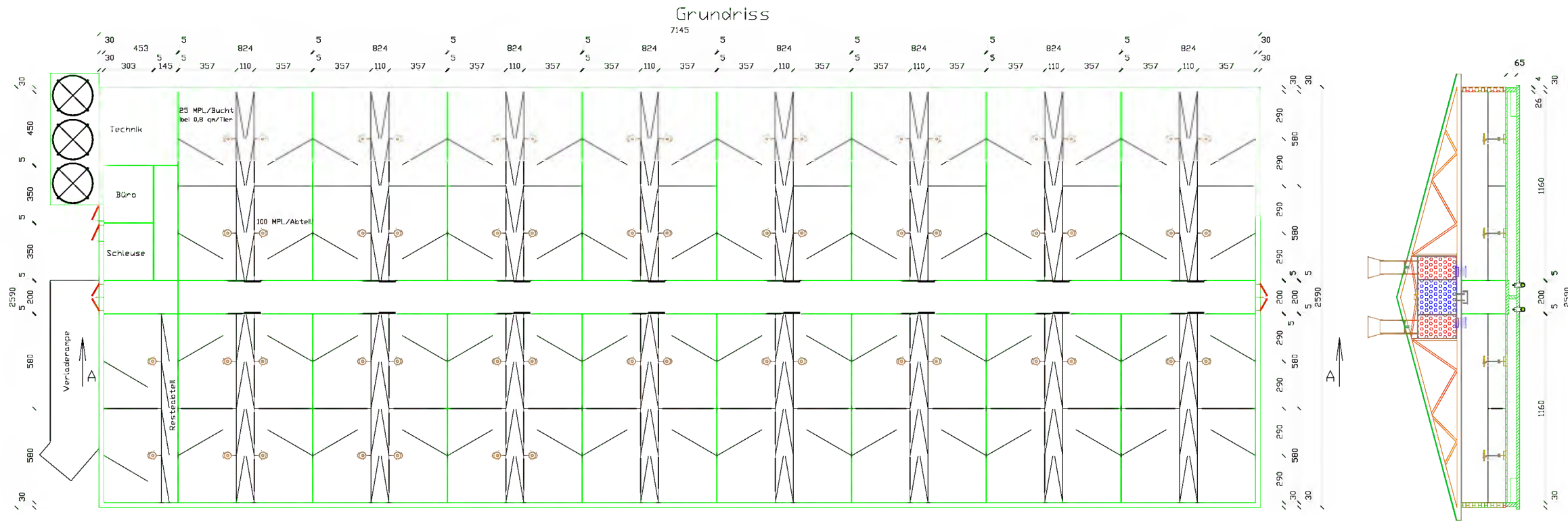
Schnitt A-A
